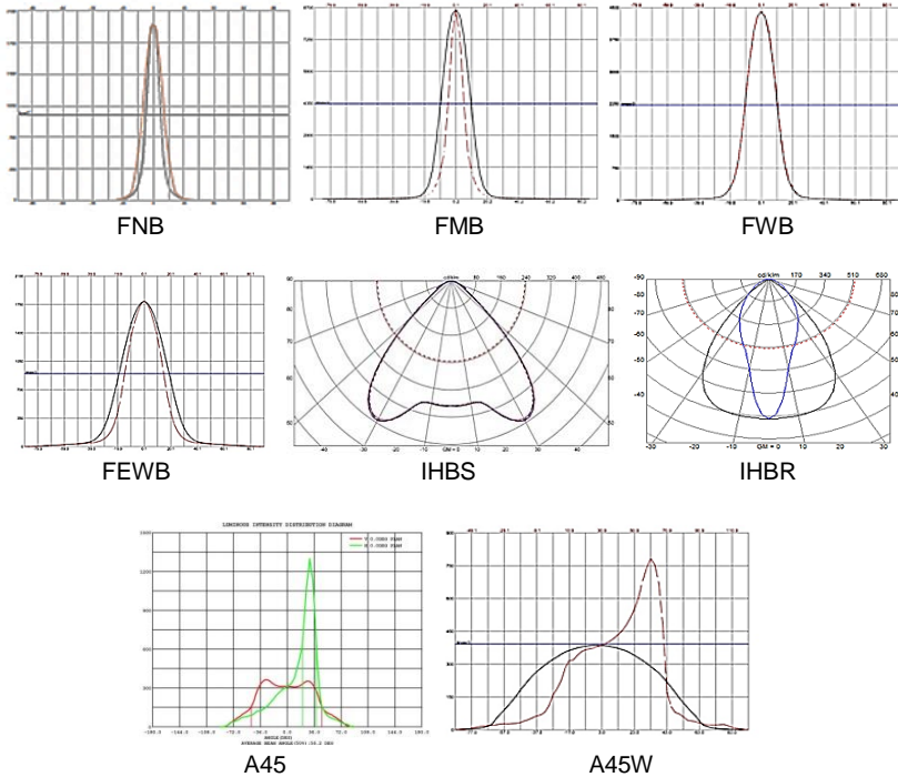
Рисунок 8.1 КСС прожектора
