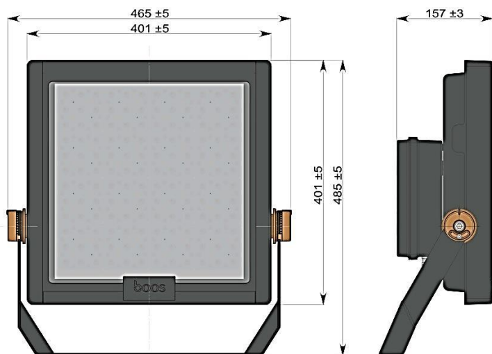
Рисунок 9.1 Габаритные размеры прожектора
